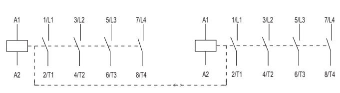
Ex9CDR... 4P 4NO
