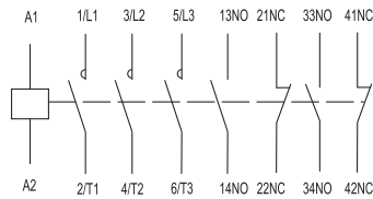
Ex9C... 3P 2NO+2NC
